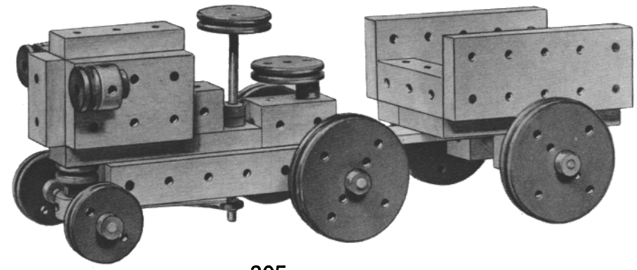
205/2 Der Traktor von unten gesehen. 205/3 Der Anhänger von unten gesehen. 205/4 Längsschnitt durch die Mitte des Traktors. 205/5 Der Traktor von der anderen Seite gesehen.
