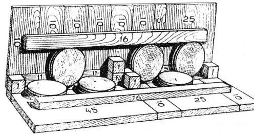
Ansicht des umgelegten Daches von Innen
