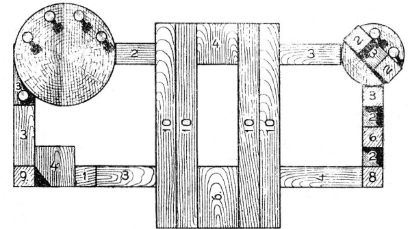
Daraufsicht des ersten Stockes in Fußbodenhöhe
