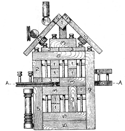
Ansicht der Seite beim Eingang
