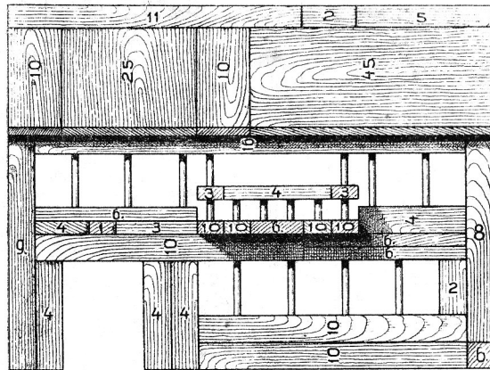
Ansicht von rückwärts
